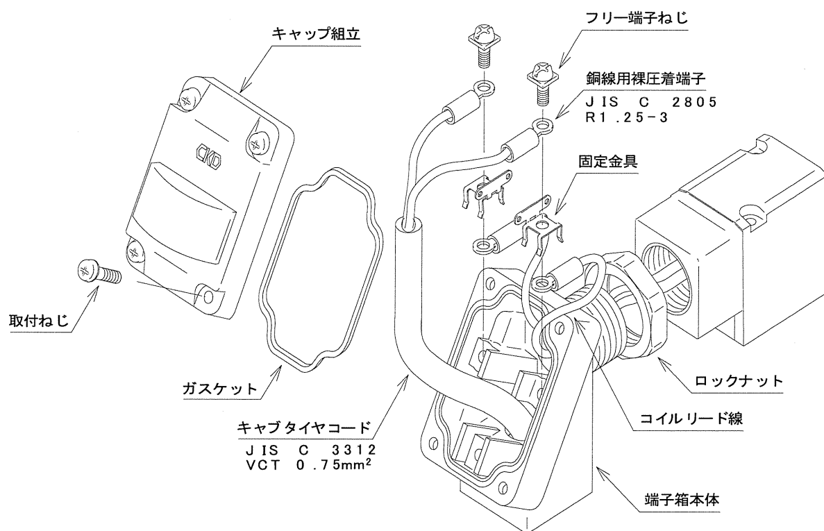
(図2-6) T型端子箱の結線方法
