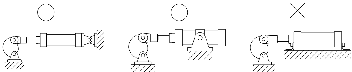
Clevis type
