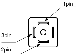
Fig. 4 DIN terminal box pin array (body side)
