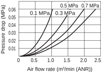
● FW8000-20-W
