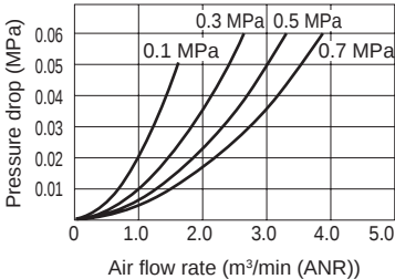
● FW8000-25-W
