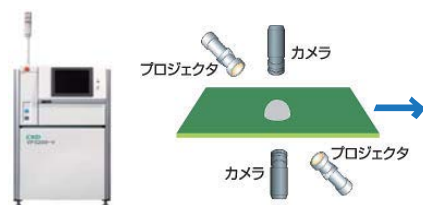
両面検査対応モデル VP5200R-V
