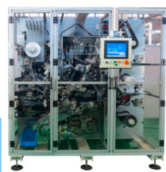
ポリマー電池用高速大型角形リチウムイオン電池捲回機
